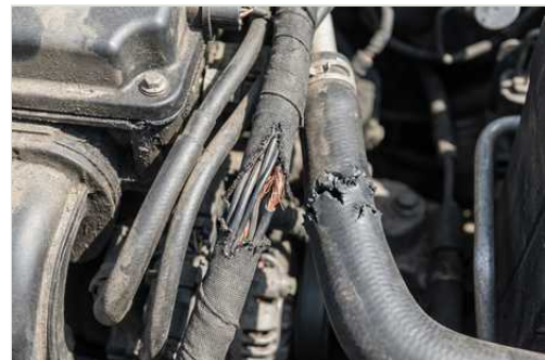
Angenagte Kabel im Motorraum sind der typische Marderschaden am Fahrzeug.
